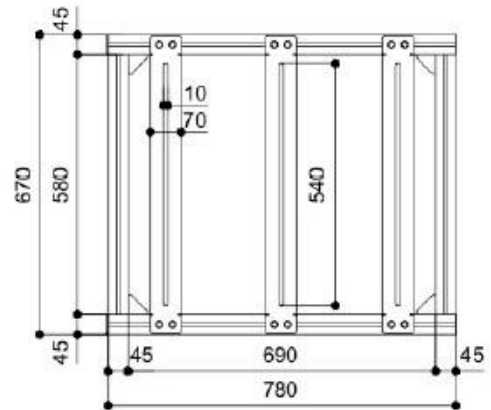
Befestigungspunkte für Projektor
