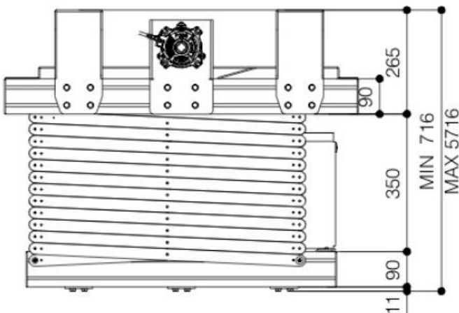
Seitenansicht – Lift geschlossen
