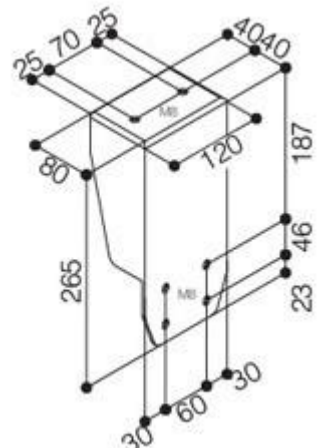
Deckenhalterung
