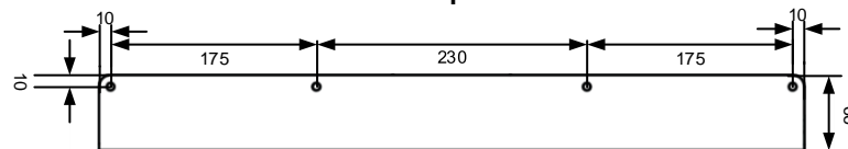
Bodenplatte Frontansicht
