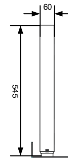
Hubsäule Seitenansicht ohne Gleitkappe
