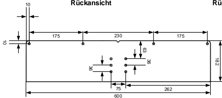
Bodenplatte
