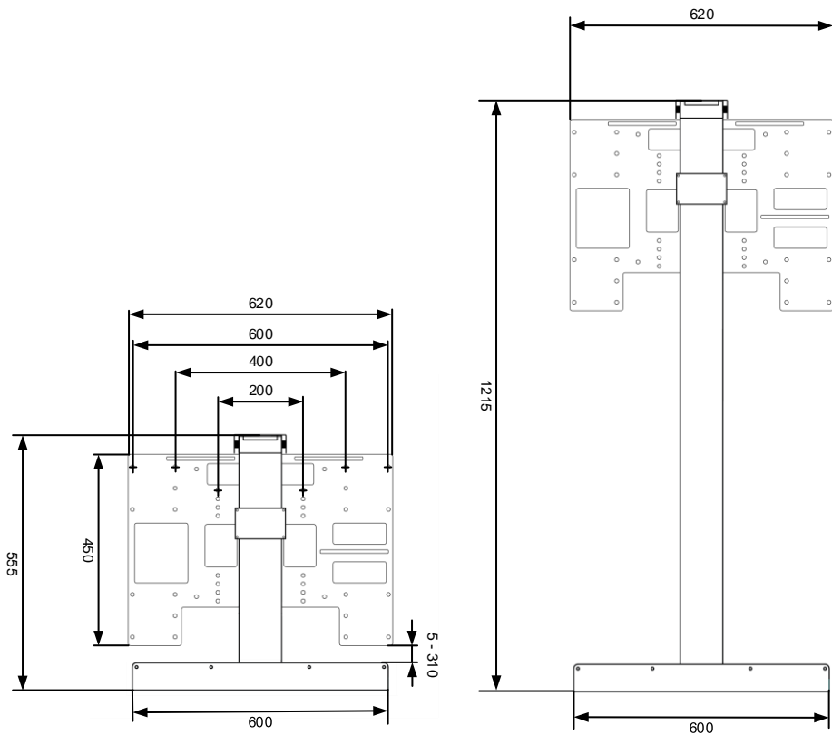
Lift Eingefahren Rückansicht
