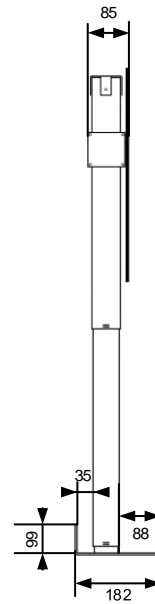
Lift Seitenansicht
