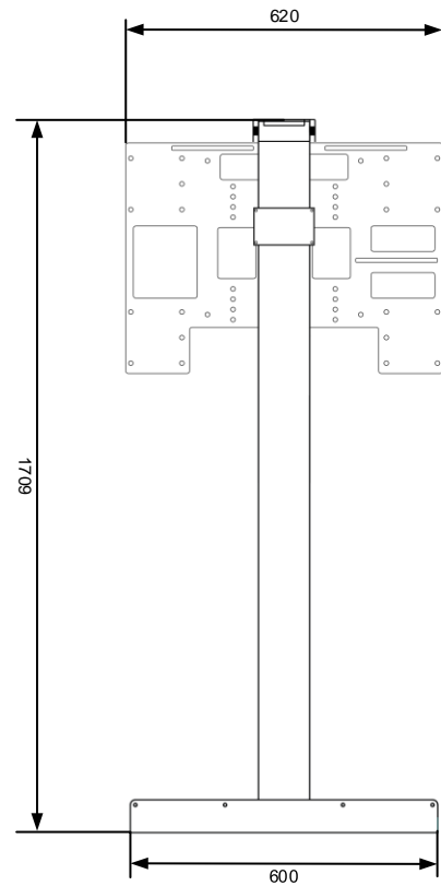
Lift Ausgefahren Rückansicht
